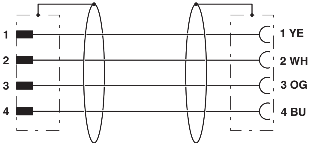
schakelschema
