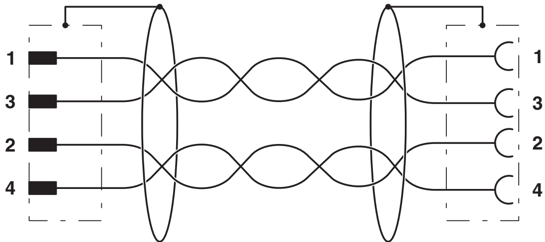
schakelschema
