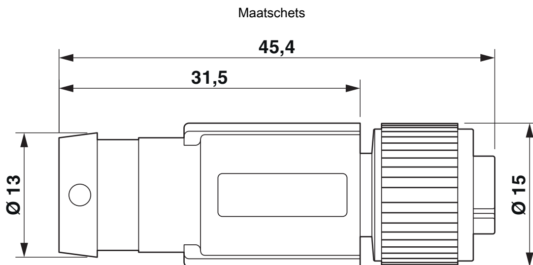
schematekening
