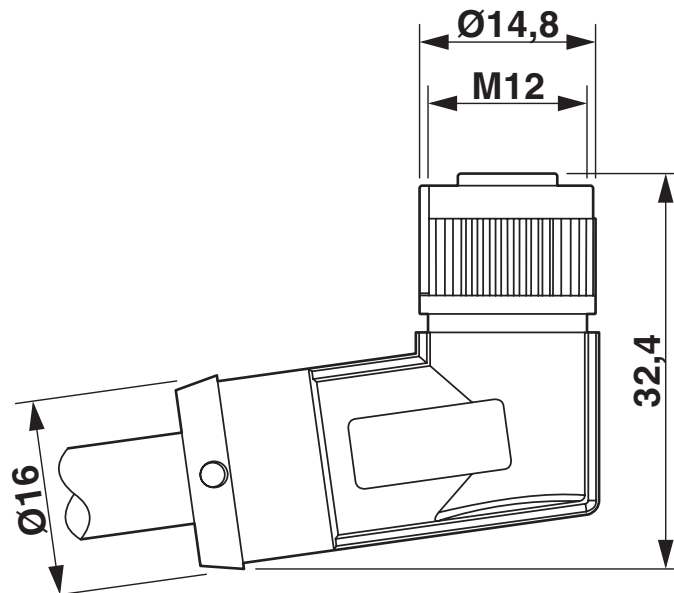
Maatschets
