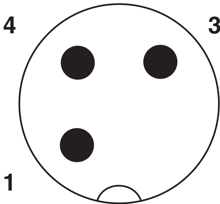
schematekening
