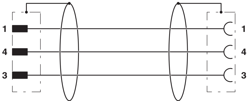
schakelschema
