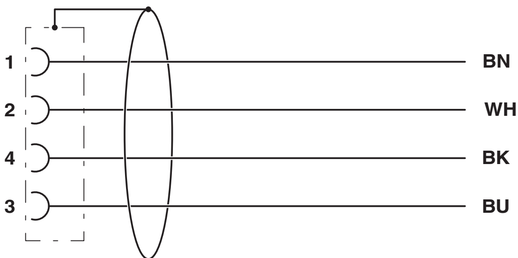
Contactbezetting van de M12-steker en de M12-bus
