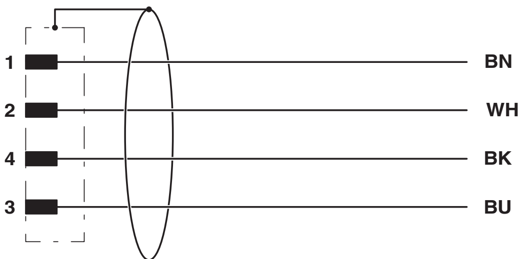
Contactbezetting van de M12-steker
