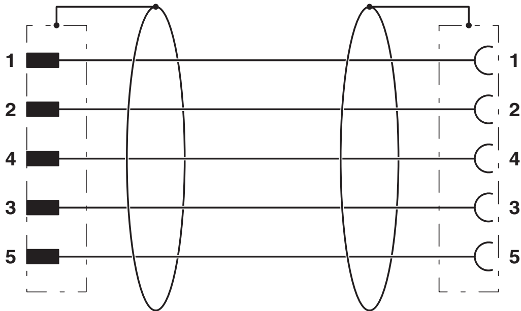
schakelschema
