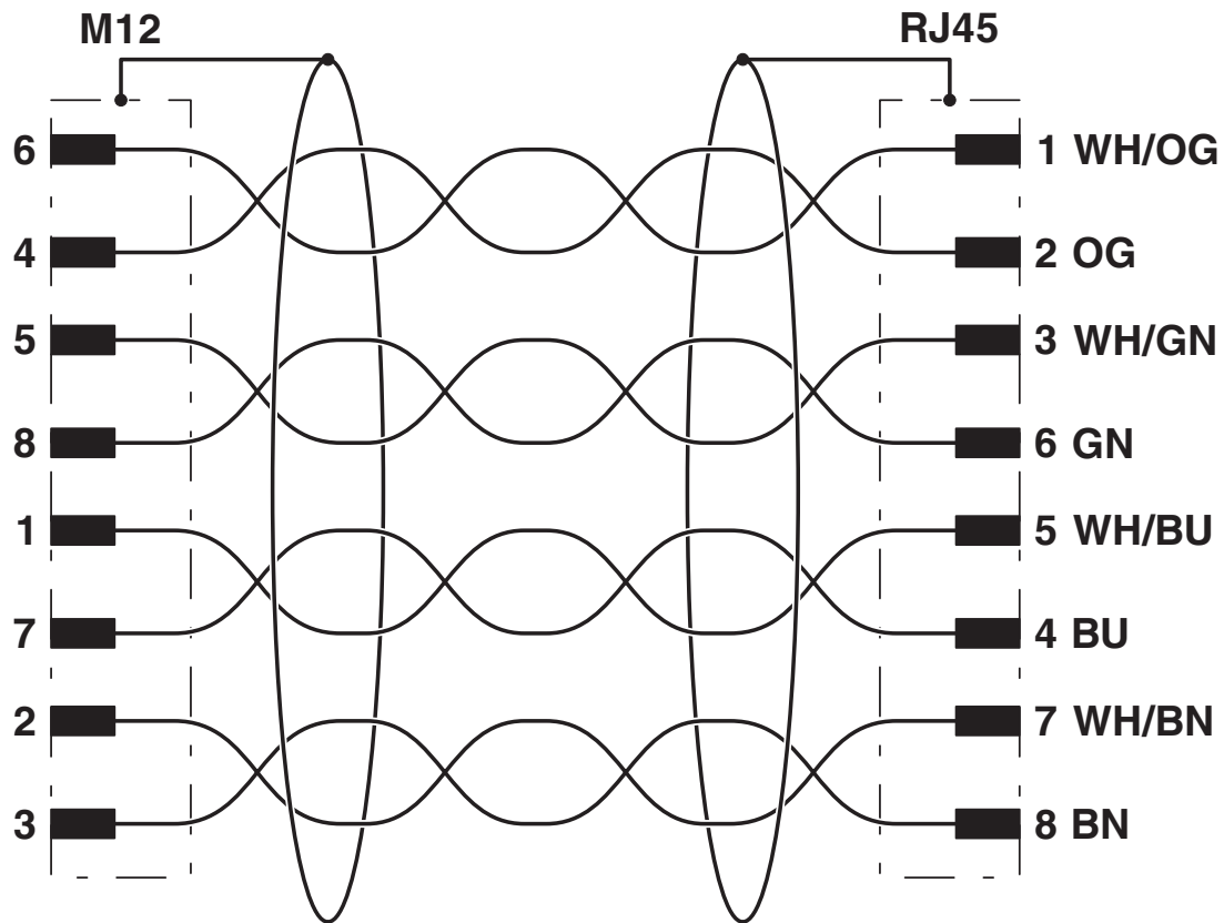
schakelschema
