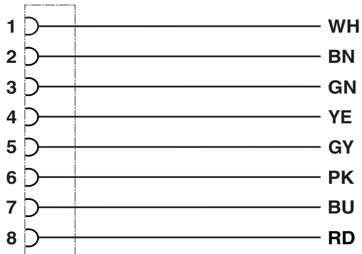
schakelschema
