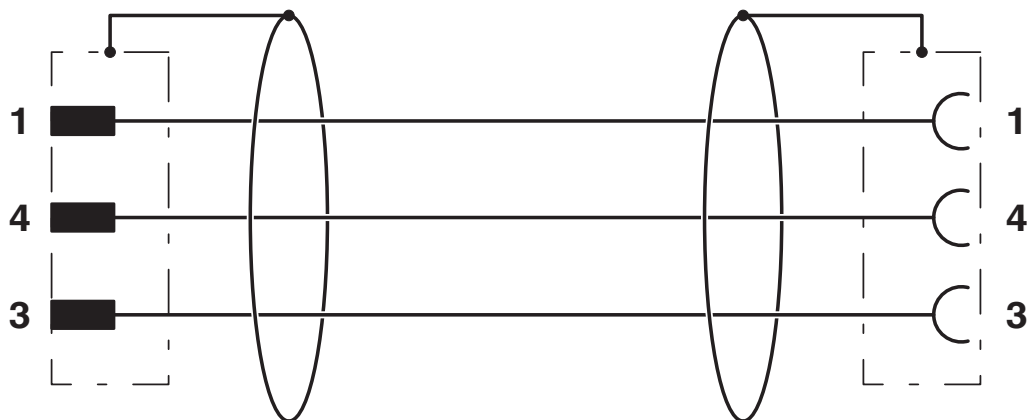
Contactbezetting van de M8-stekers/-bussen
