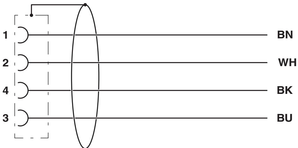
Contactbezetting van de M8-bus
