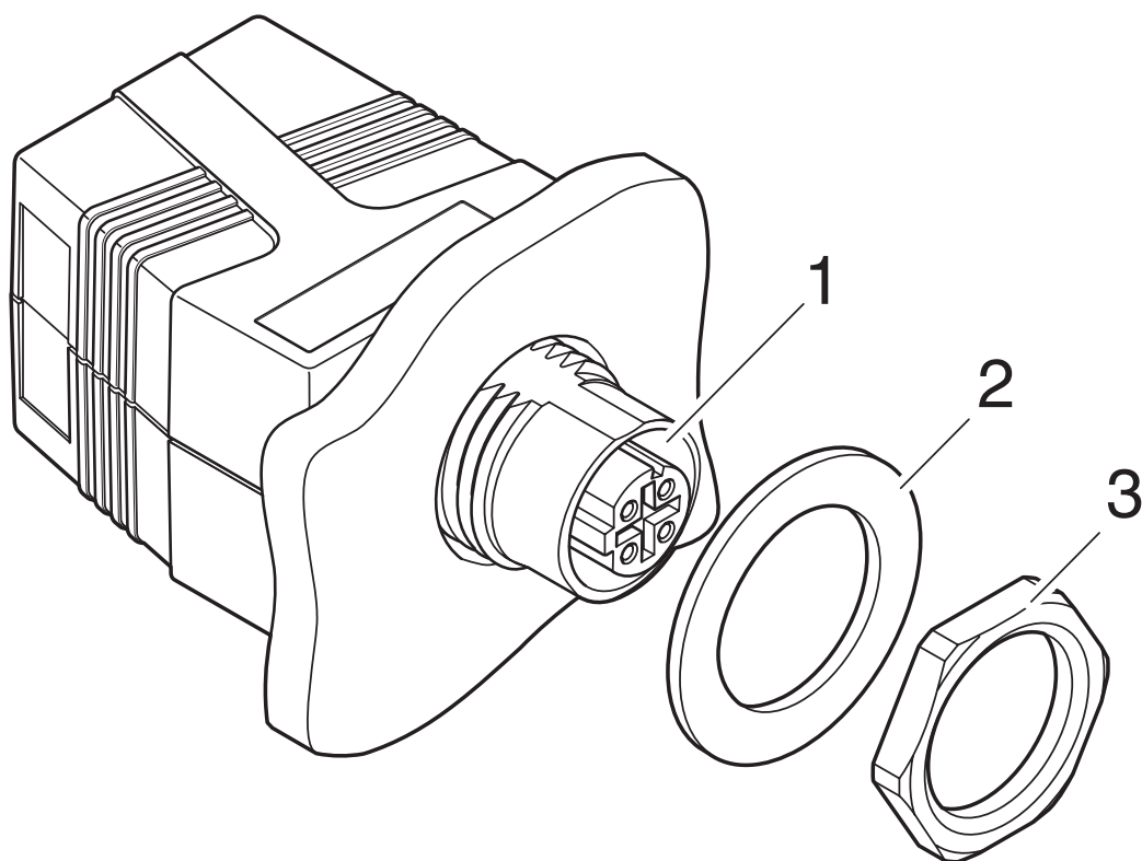
detailtekening
