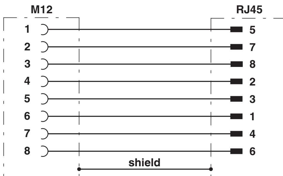
schakelschema
