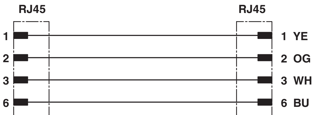
schakelschema
