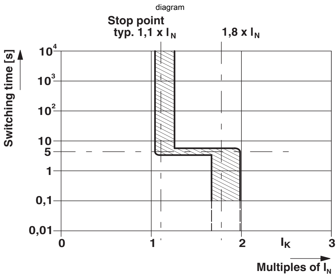
Uitschakelkarakteristiek
