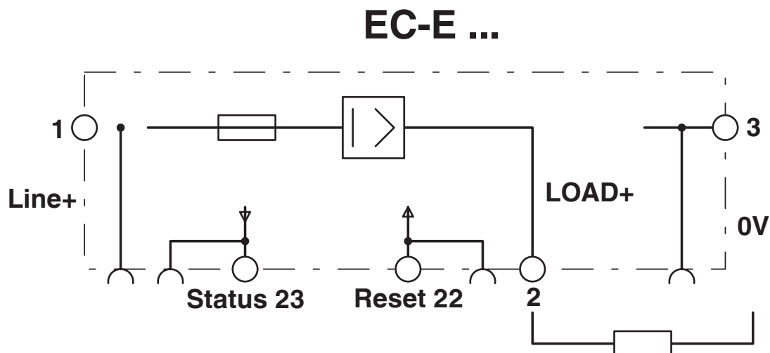
schakelschema
