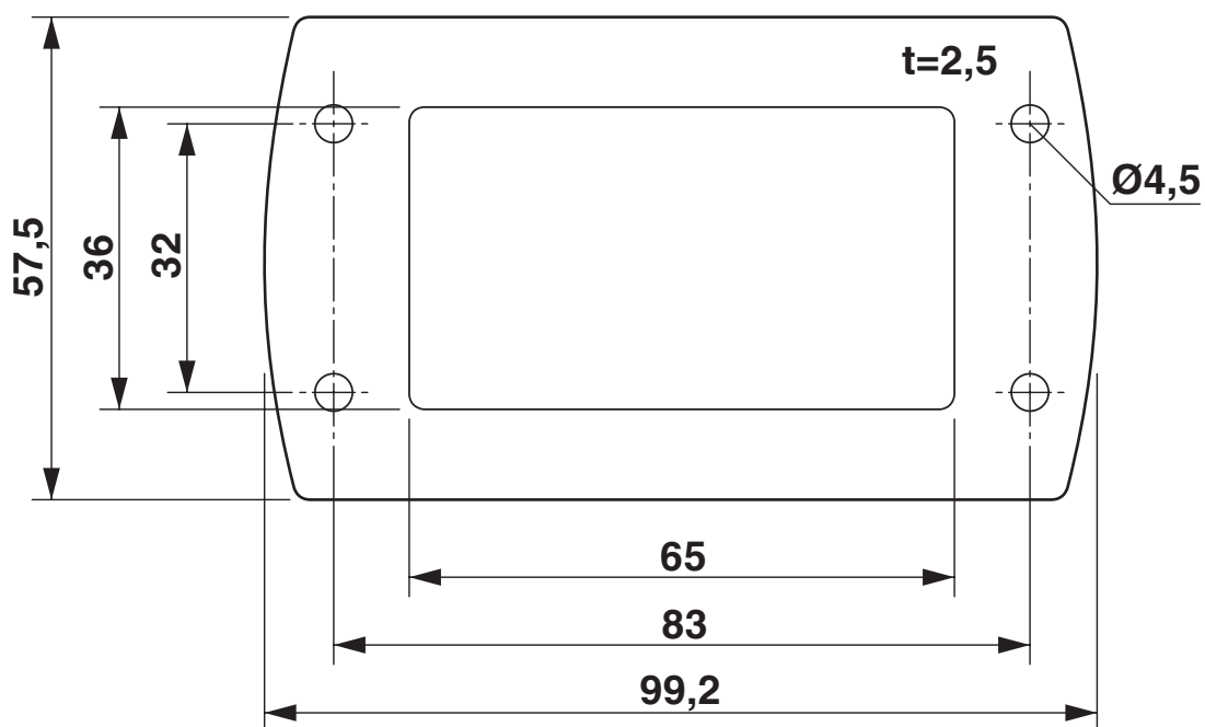
Maatschets
