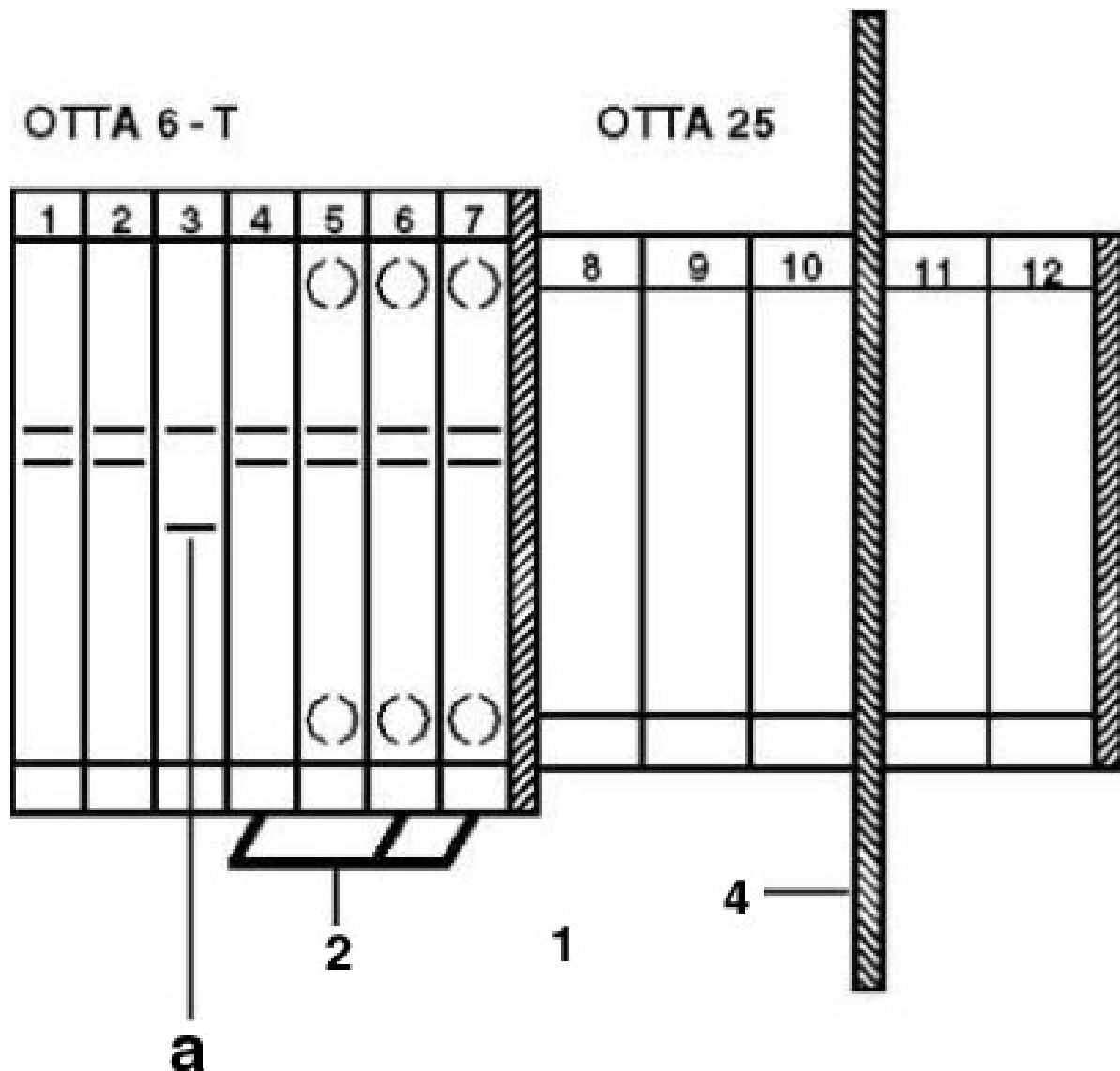
schakelschema
