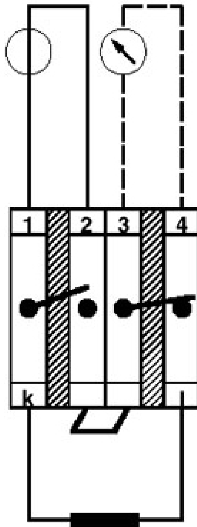
schematekening
