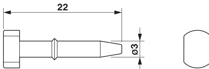
外形寸法
