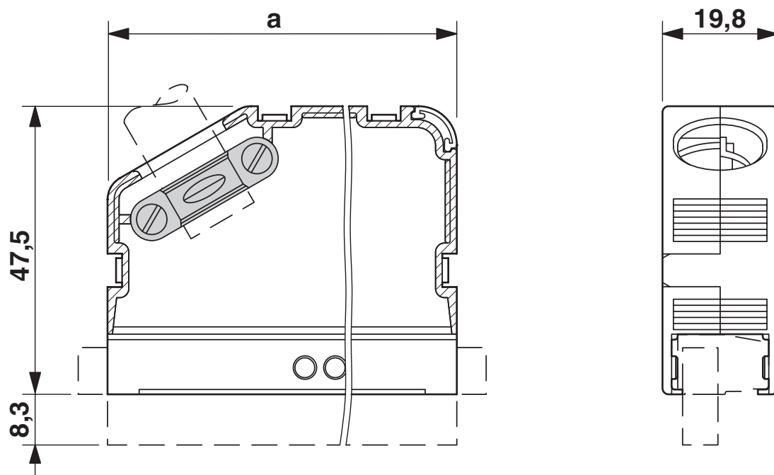
外形寸法
