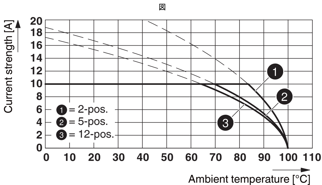
型式 : FRONT-MSTB 2,5/...-STとMDSTBV 2,5/...-Gの組合せ
