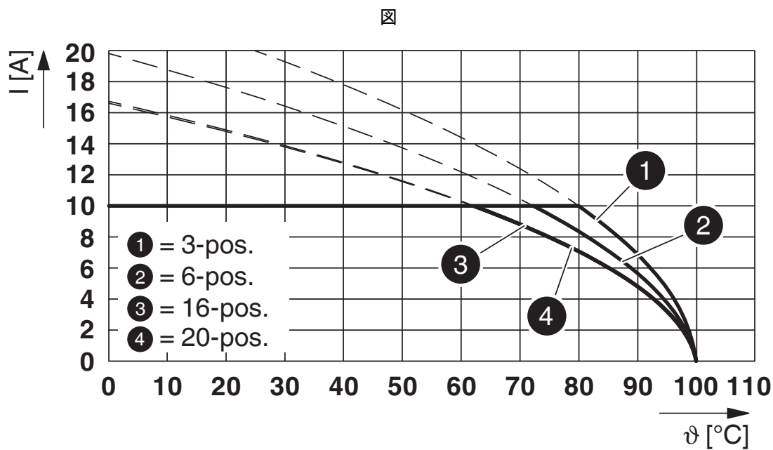
型式 : FRONT-MSTB 2,5/...-STとMDSTBV 2,5/...-G1の組合せ
