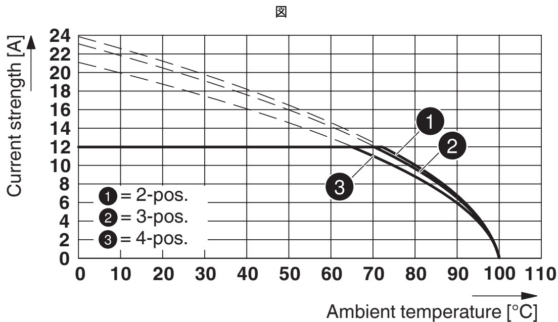
型式 : FRONT-MSTB 2,5/...-STとMSTBO 2,5/...-G1Lの組合せ
