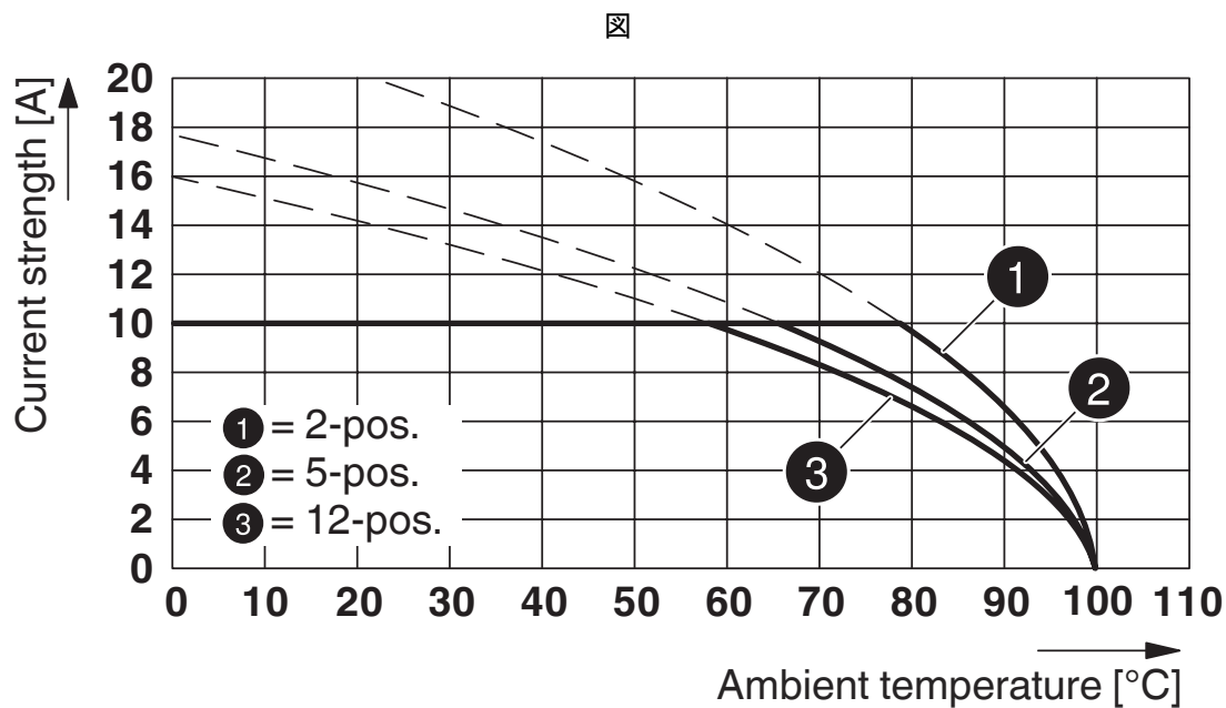
型式 : FRONT-MSTB 2,5/...-STとMDSTBA 2,5/...-Gの組合せ
