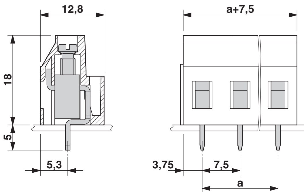
外形寸法
