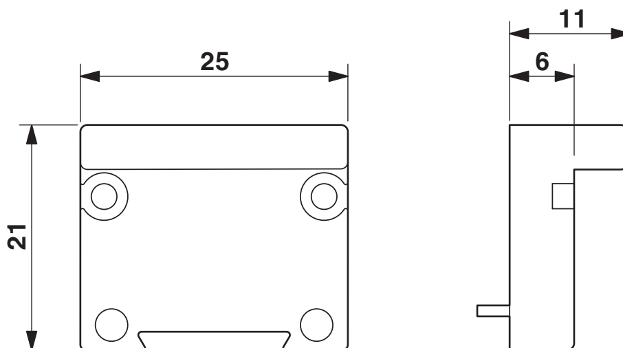
Disegno quotato
