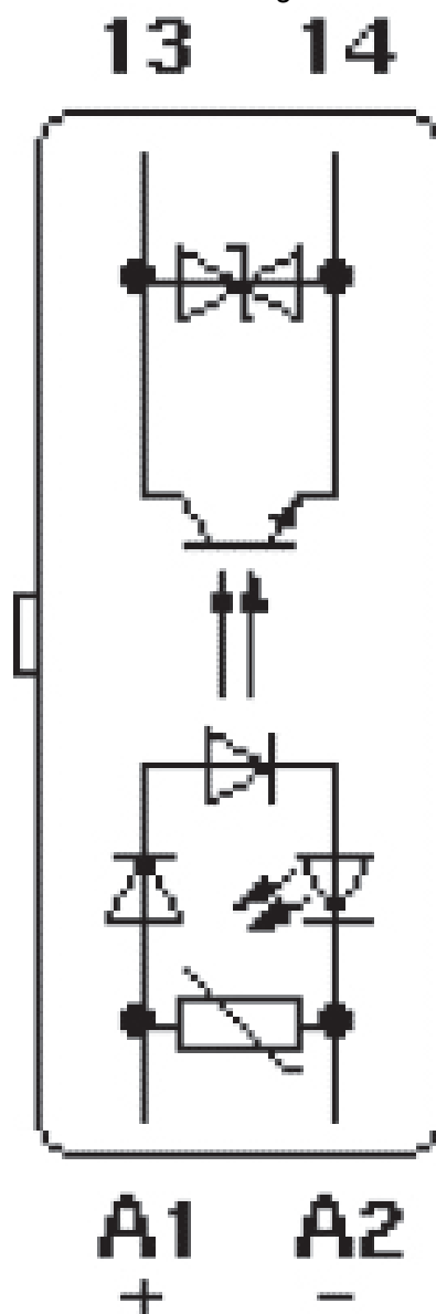
Schema di collegamento
