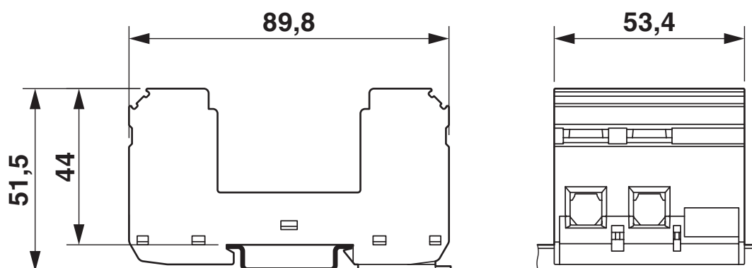
Disegno quotato
