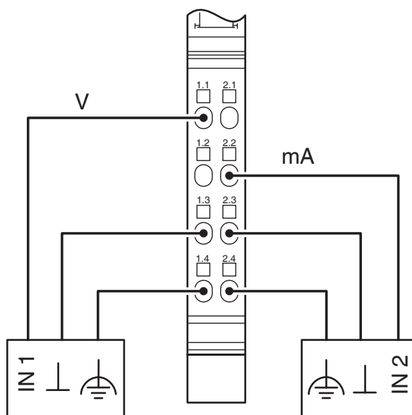
Disegno collegamento
