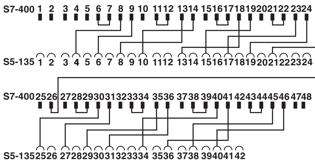
Schema di collegamento FLKM S135-460-4UA/I/S400
