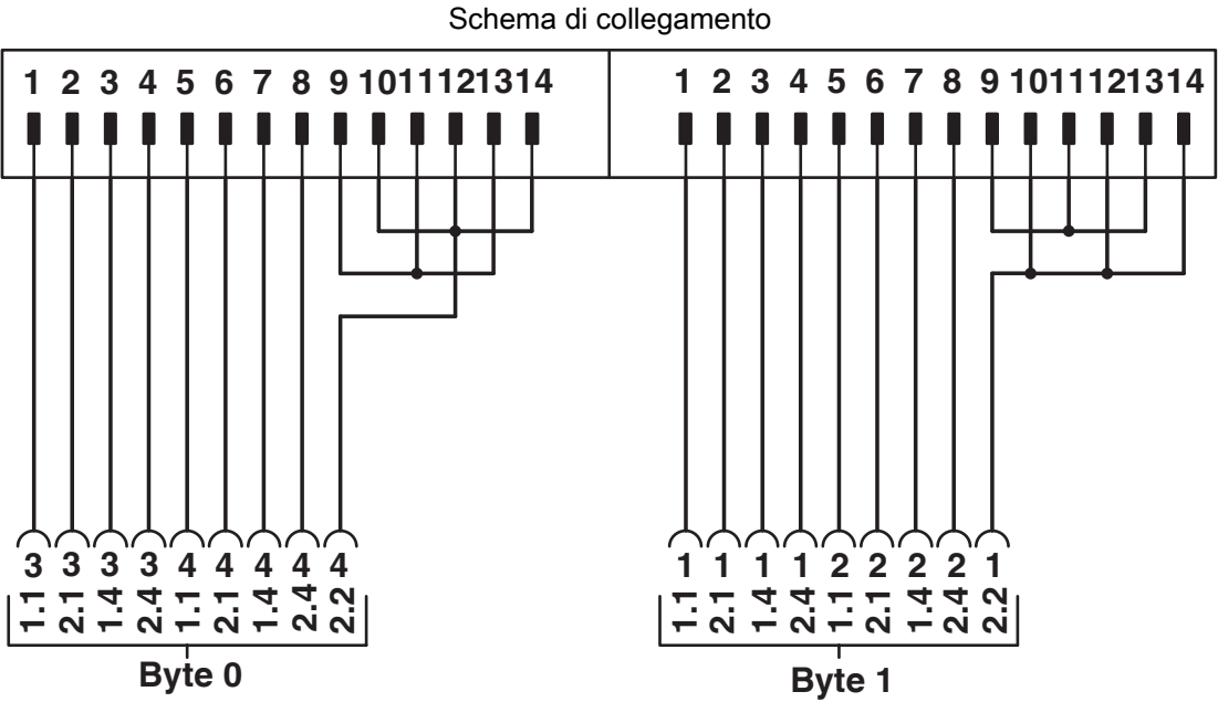
Schema di collegamento FLKM 14-PA-INLINE/OUT16
