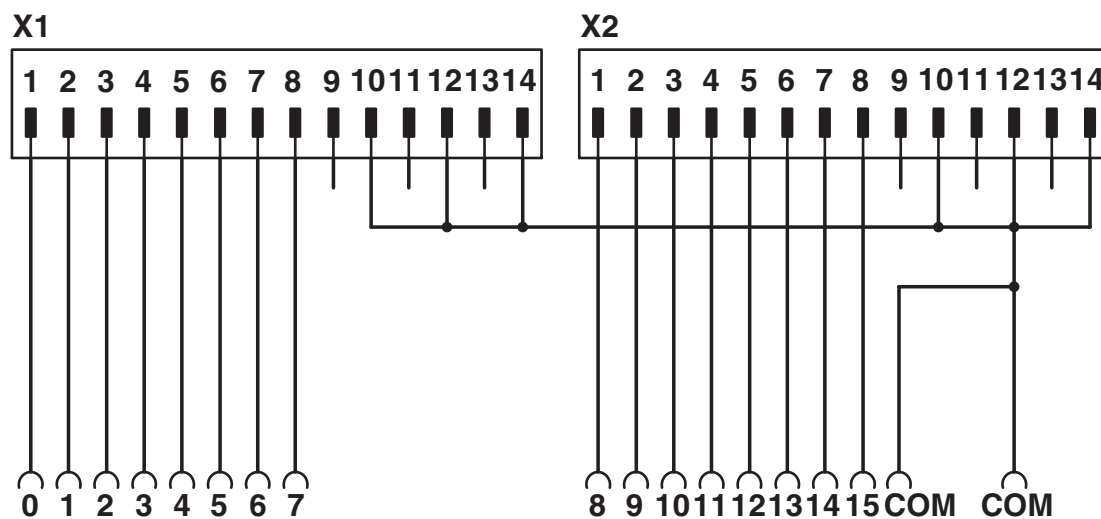
Schema di collegamento FLKM 14-PA-SLC500/IN
