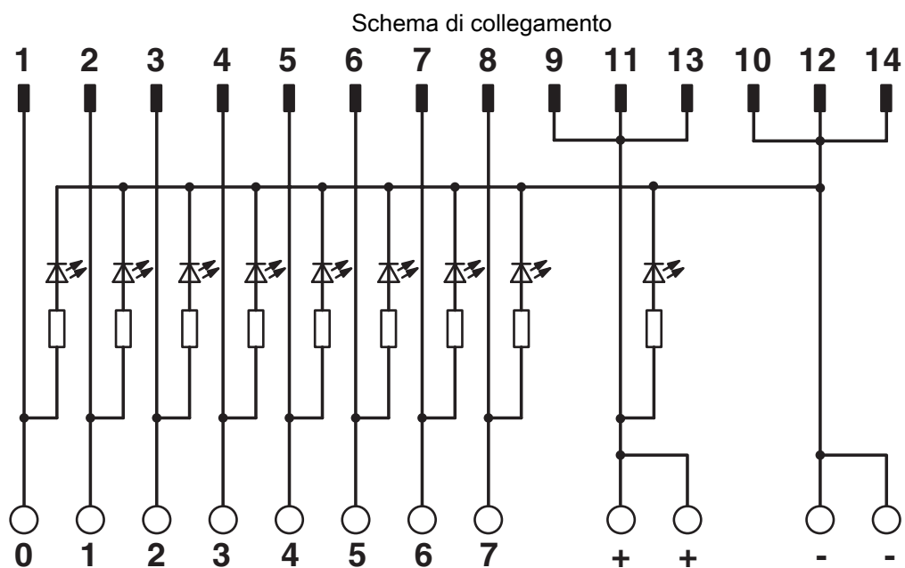
Schema di collegamento FLKM 14/LA/PLC
