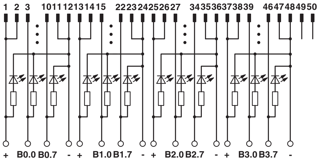
Schema di collegamento FLKM 50/LA/PLC
