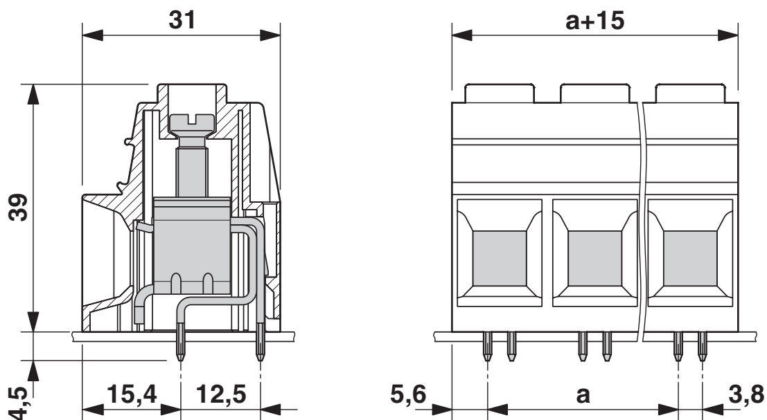
Disegno quotato
