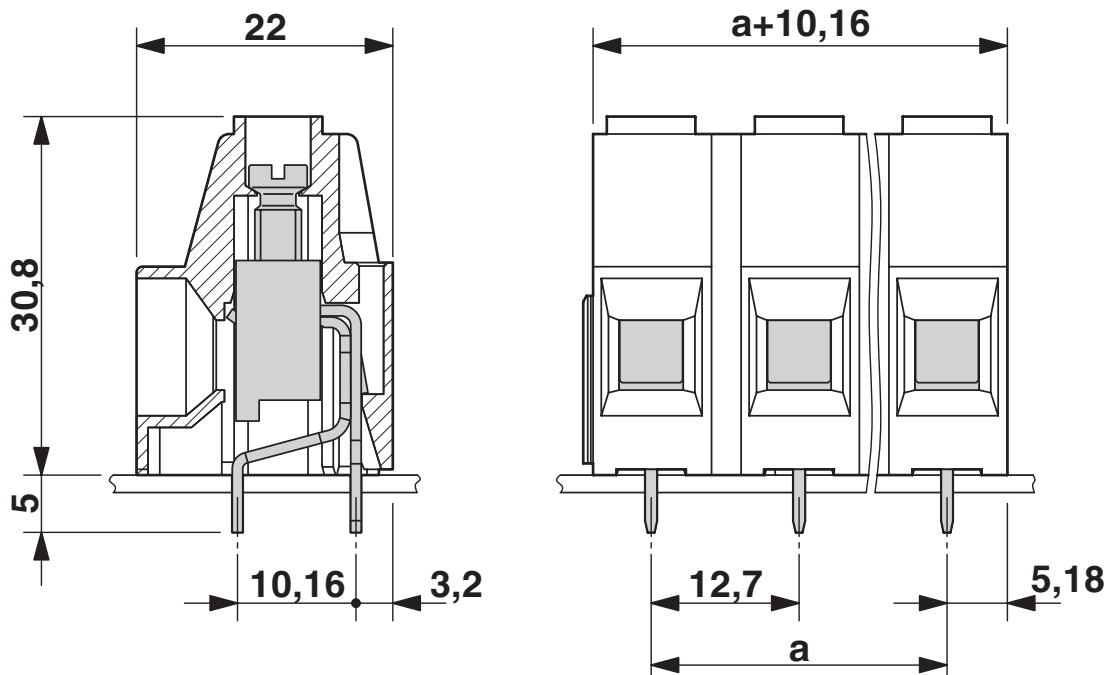
Disegno quotato
