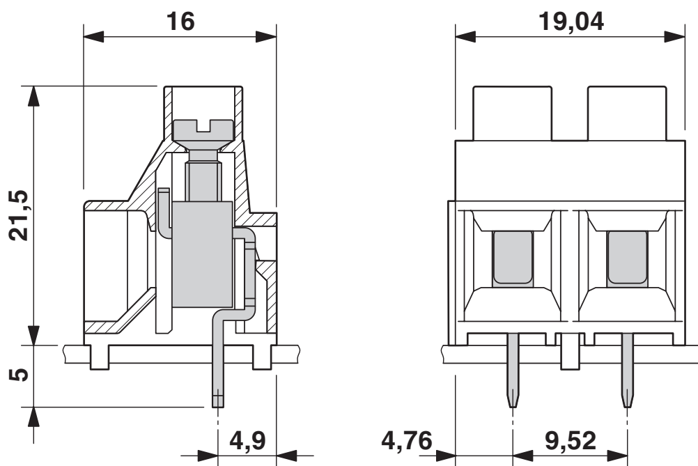
Disegno quotato
