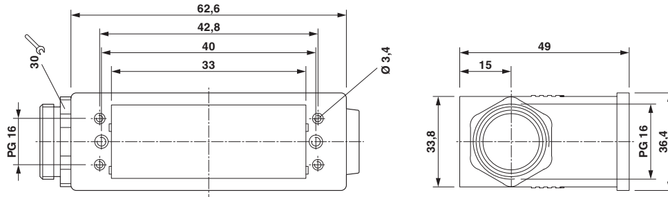
Disegno quotato
