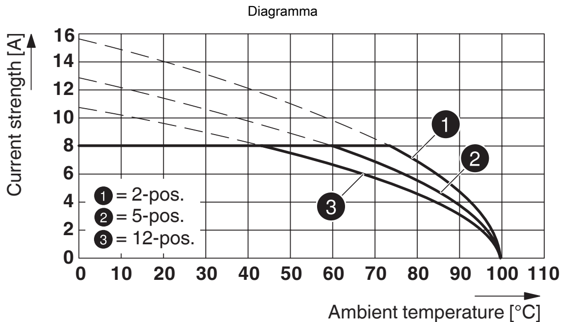
Tipo: MCVW 1,5/...-ST-3,5 AU con MCV 1,5/...-G-3,5 AU
