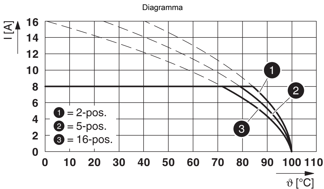
Tipo: FMC 1,5/...-ST-3,5 AU con MCV 1,5/...-G-3,5 AU
