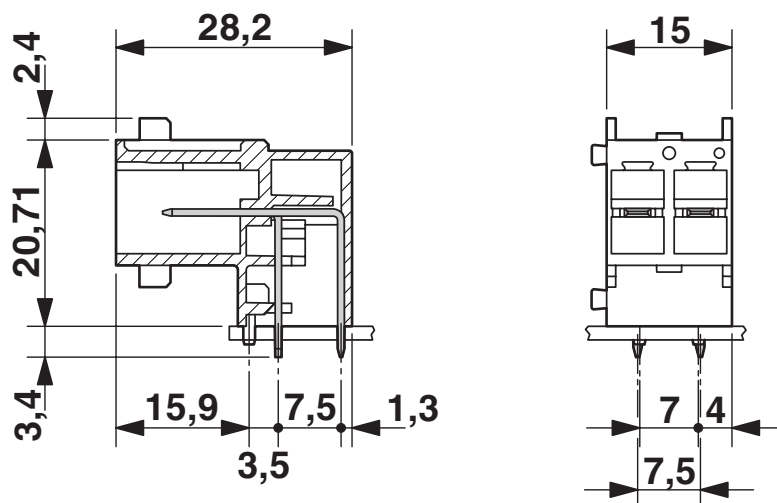
Disegno quotato
