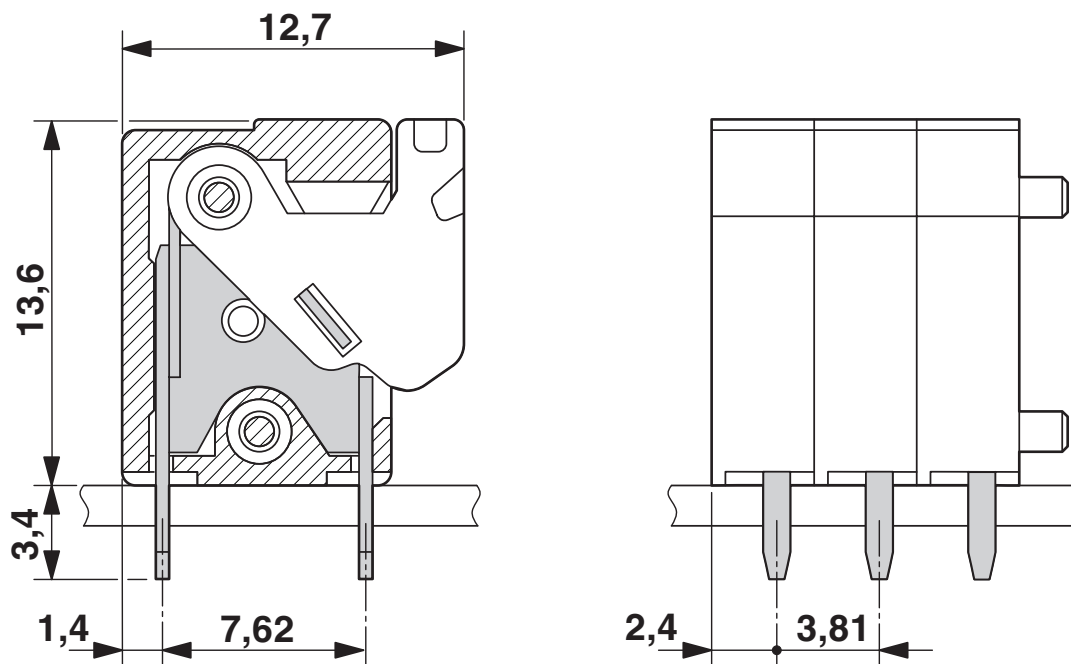
Disegno quotato
