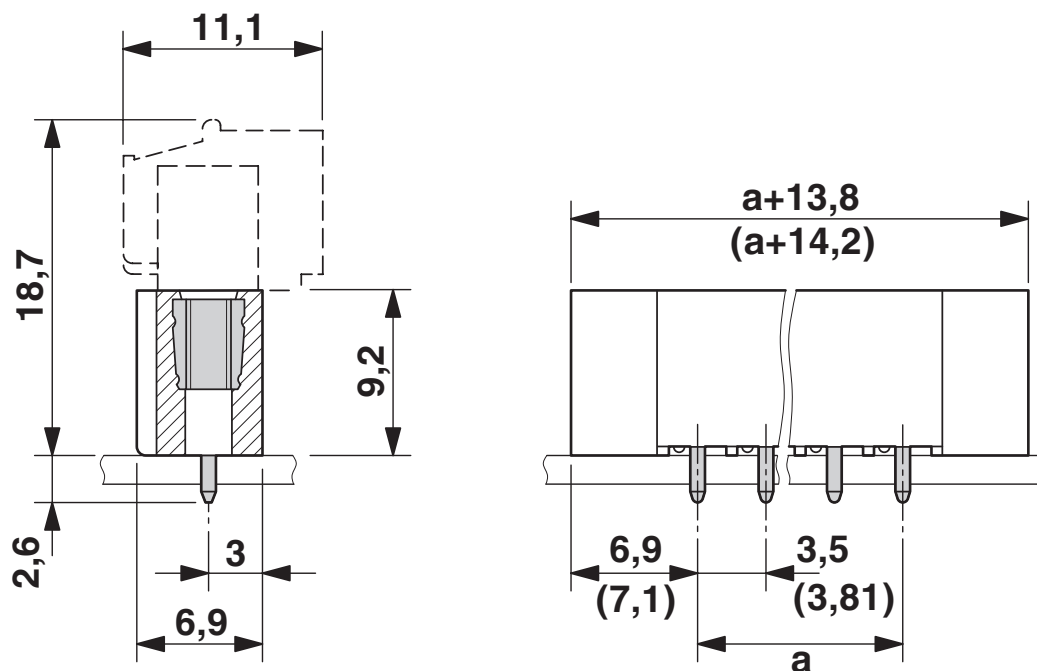
Disegno quotato
