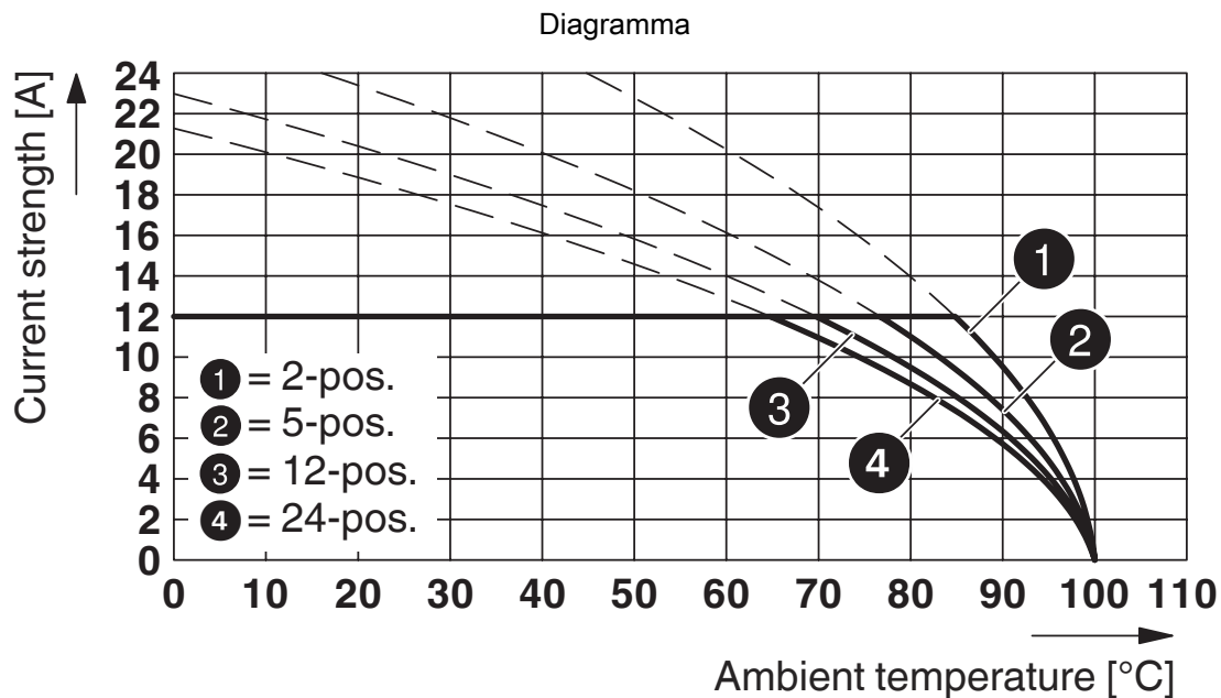
Tipo: MSTB 2,5/...-ST con CCA 2,5/10-ST
