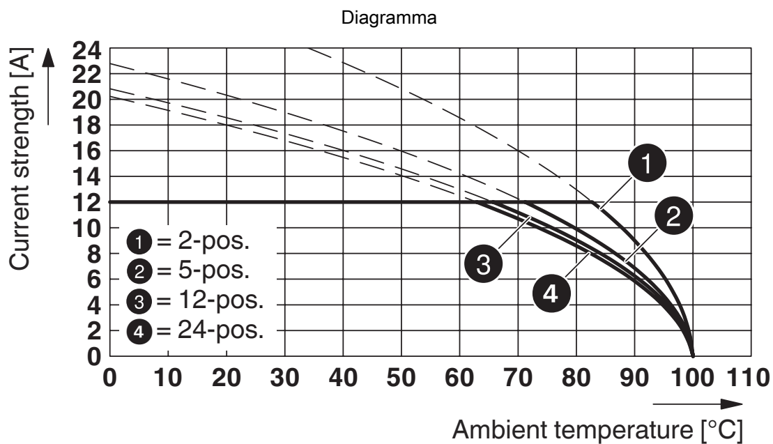
Tipo: MSTB 2,5/...-ST con CCVA 2,5/10-ST
