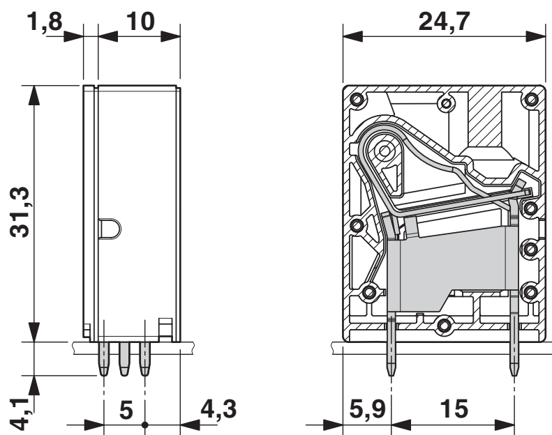
Disegno quotato
