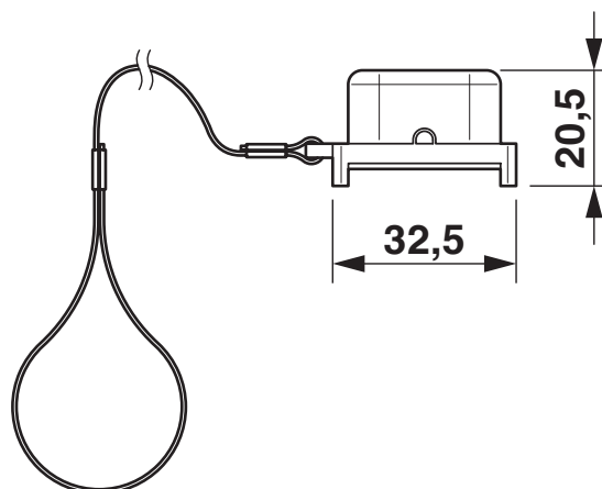
Disegno quotato
