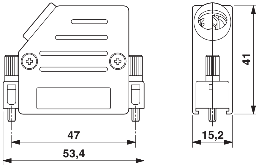
Disegno quotato
