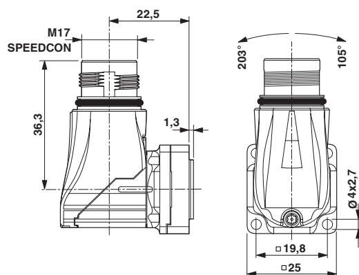
Disegno quotato
