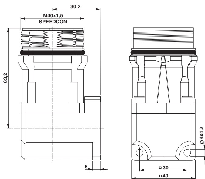
Disegno quotato
