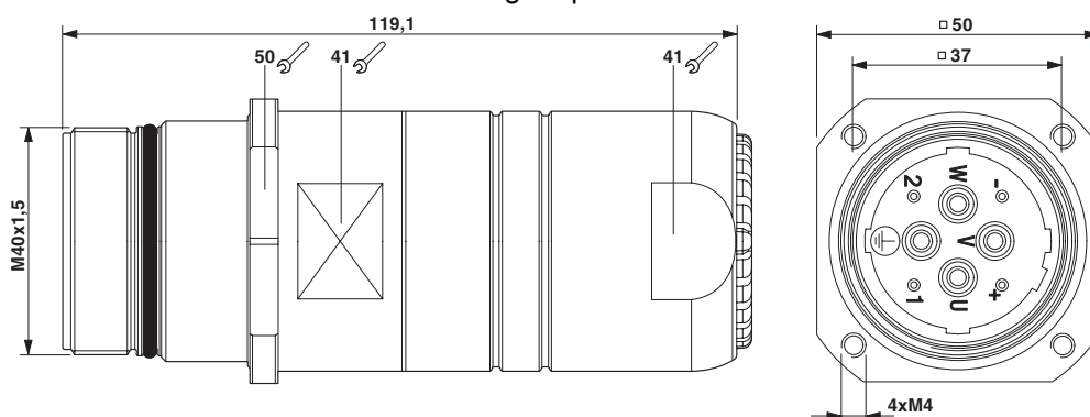
Disegno quotato
