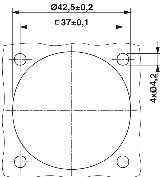
Disegno quotato
