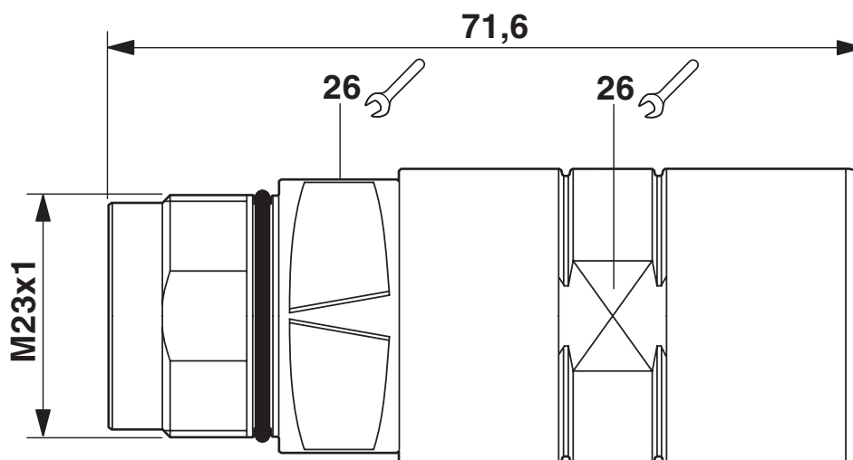
Disegno quotato
