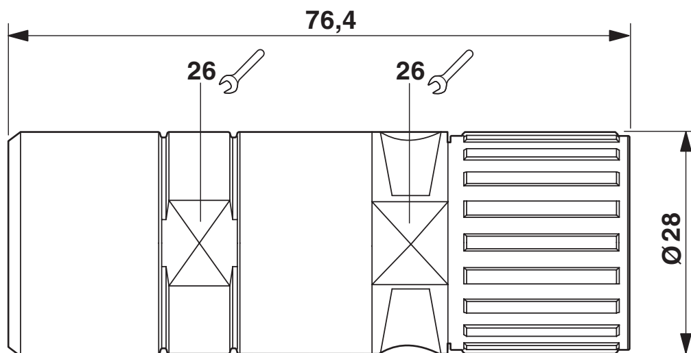
Disegno quotato
