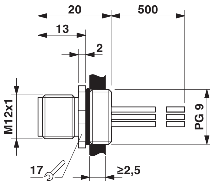
Disegno quotato
