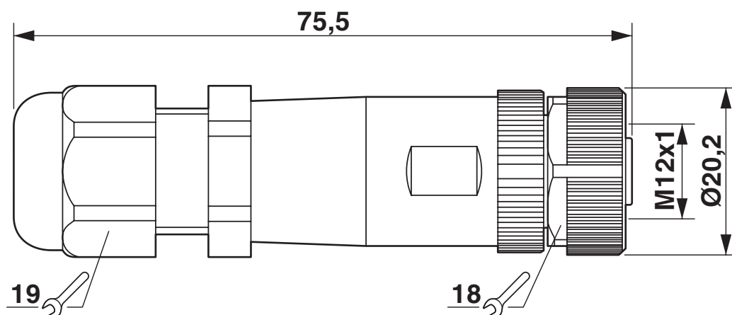
Disegno quotato
